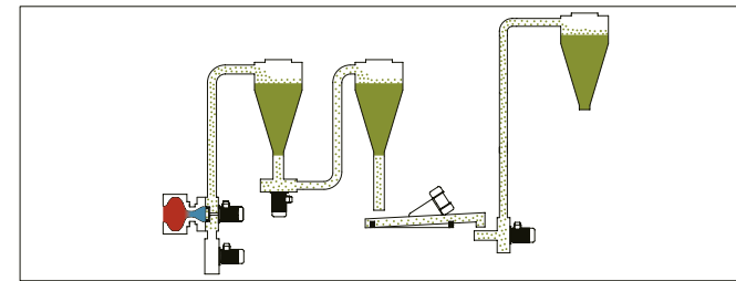
Hava Soğutmalı Sıcak Hava Kafadan Kesme Peletleme Sistemi
