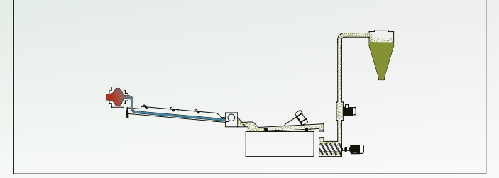
Otomatik Makarna Kesim Peletleme Sistemi
