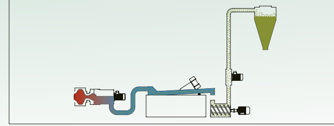
Su Halkası Peletleme Sistemi
