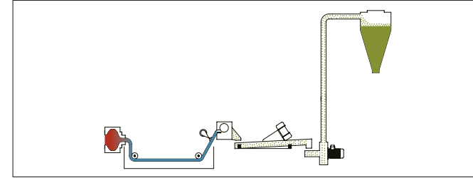
Su Soğutmalı Makarna Kesim Peletleme Sistemi
