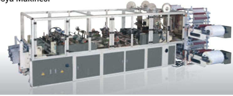
MGA-40A-400 Yüksek Hızlı ClearHolder(E310) Makinesi
