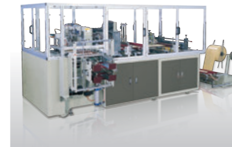
MGA-56-700 Tam Otomatik Ayrıştırma ve Kesme Makinesi
